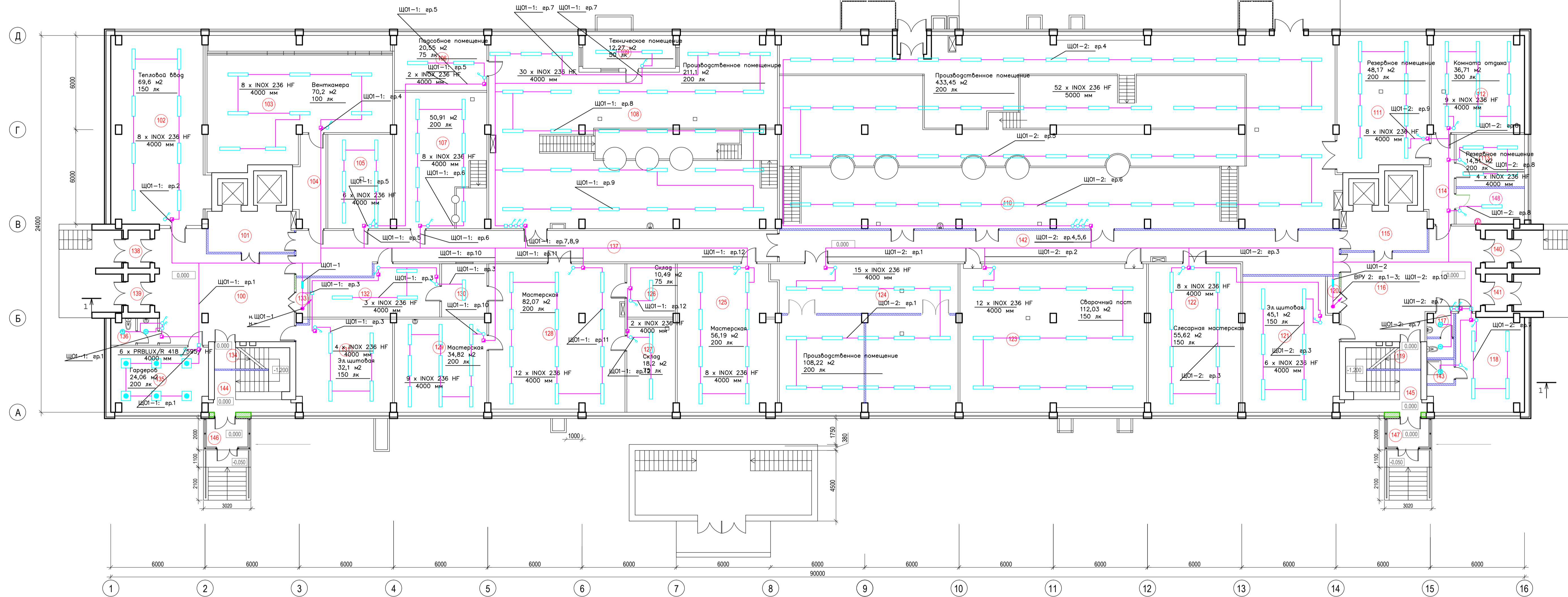
Экспликация помещений
