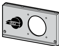
FMCE 48 2CMA191085R1000 1 ряд 1 место Крышка для установки одного разъема с блокировочным выключателем, 16 А
