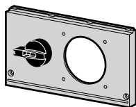
FMCE 49 2CMA191086R1000 1 ряд 1 место Крышка для установки одного разъема с блокировочным выключателем, 32 А
